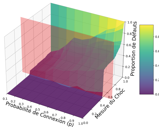
Figure 4: Surface 3D illustrant la relation entre la densité du réseau, l'amplitude du choc et la proportion de défauts résultante.
